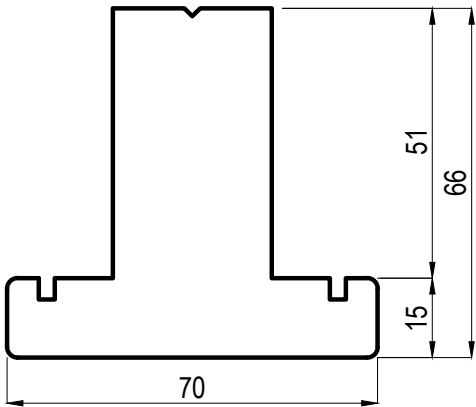
FD633T Tecnorovere Predisposizione per montaggio guarnizione DE132DN
