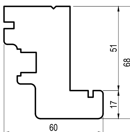
FD613T Tecnorovere Predisposizione per montaggio guarnizione DE132DN
