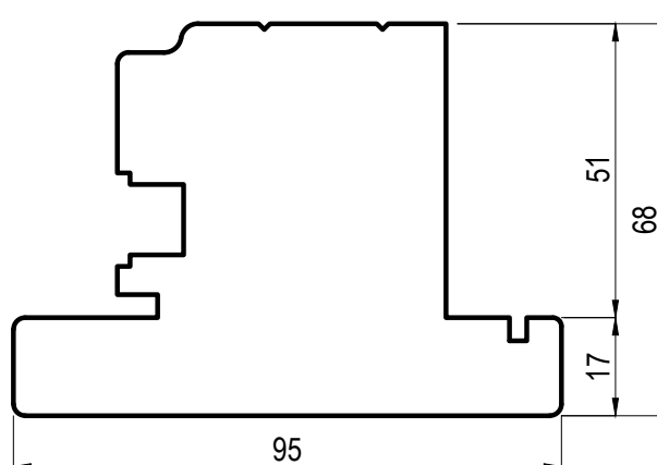
FD614T Tecnorovere Predisposizione per montaggio guarnizione DE132DN
