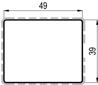
FD642N Pino lamellare rivestito FD642P Pino lamellare grezzo FD642T Tecnorovere
