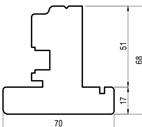
FD611T Tecnorovere Predisposizione per montaggio guarnizione DE132DN
