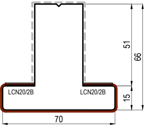
FD634N Pino lamellare rivestito FD634P Pino lamellare grezzo FD634T Tecnorovere
