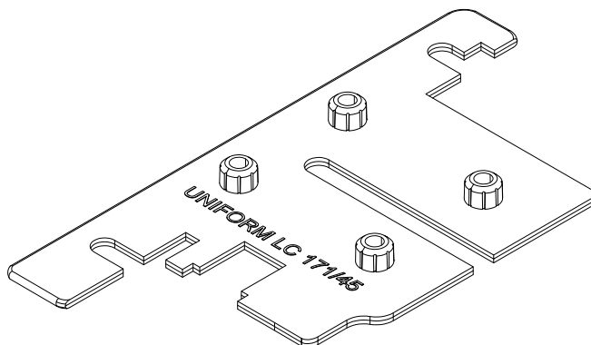
LC171-45 Accessorio giunzione 45° per FD614
