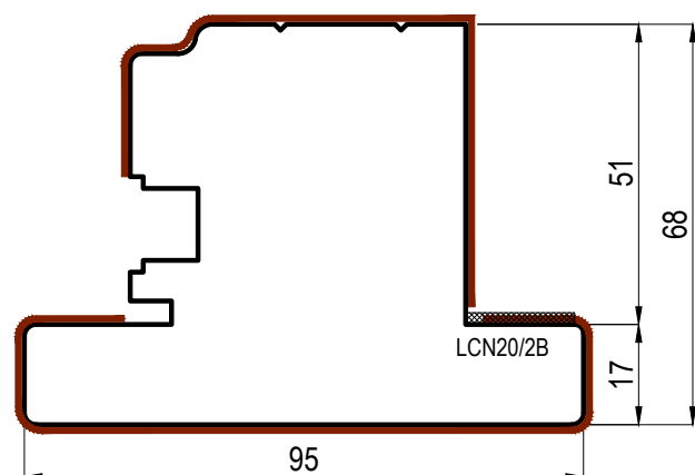
FD613N Pino lamellare rivestito Con nastro strutturale pre montato
