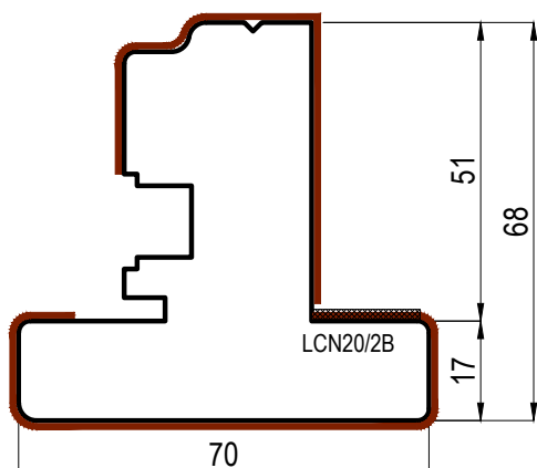
FD614N Pino lamellare rivestito Con nastro strutturale pre montato
