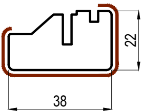
FD634N Pino lamellare rivestito FD634P Pino lamellare grezzo FD634T Tecnorovere
