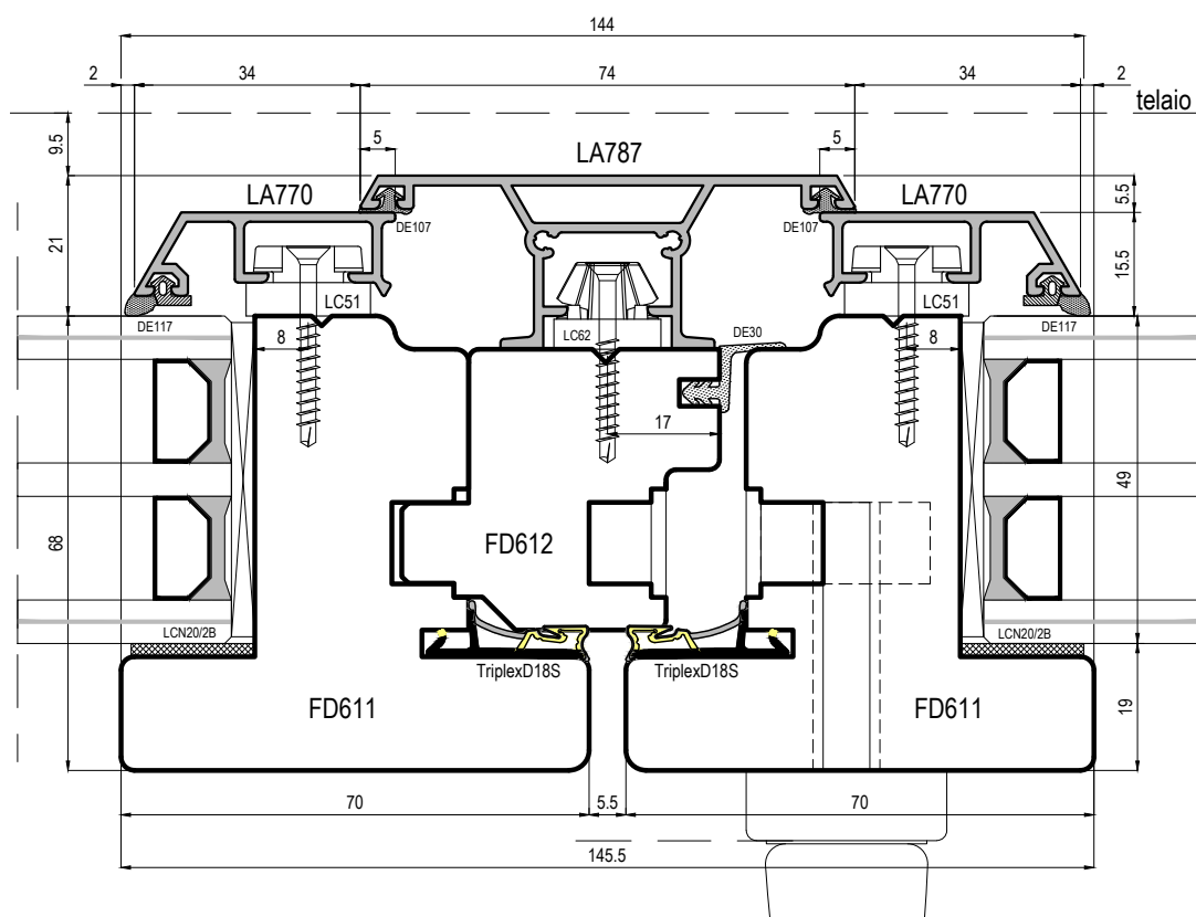
Sezione chiusura centrale porta
