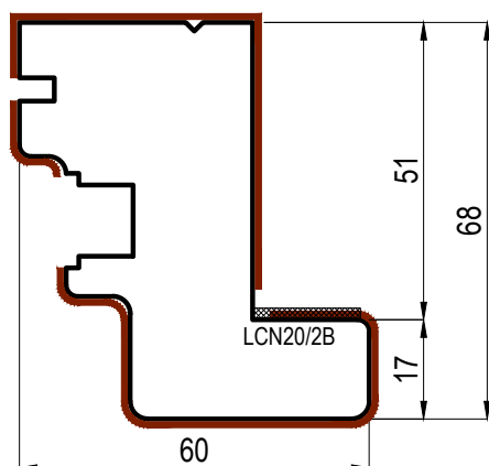
FD613N Pino lamellare rivestito Con nastro strutturale pre montato
