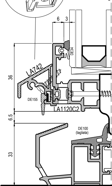
Variante con grondalino
