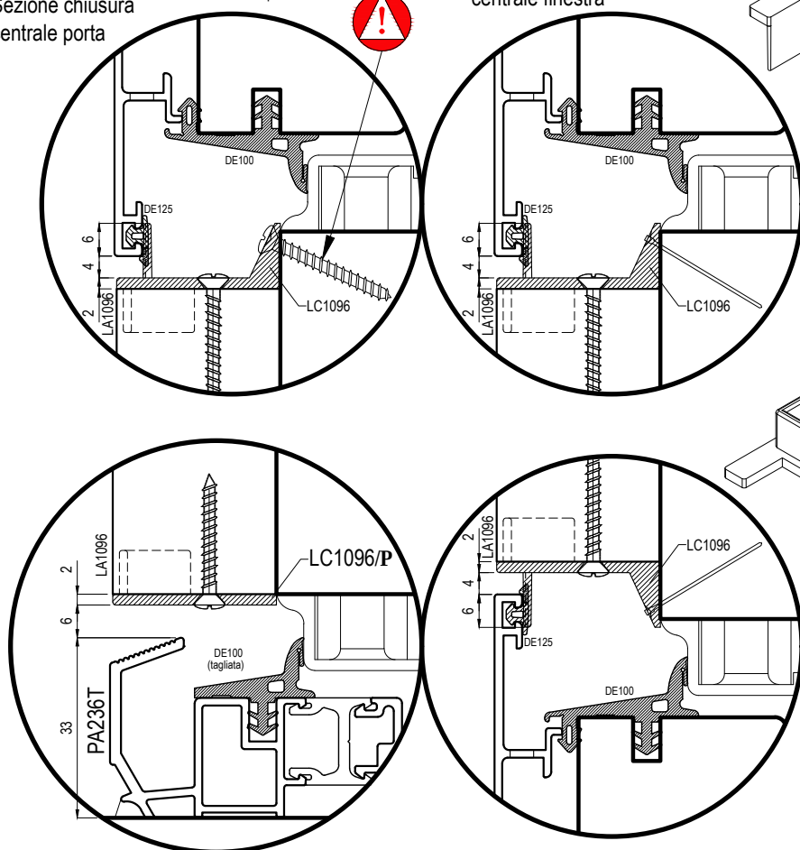
Sezione chiusura centrale finestra
