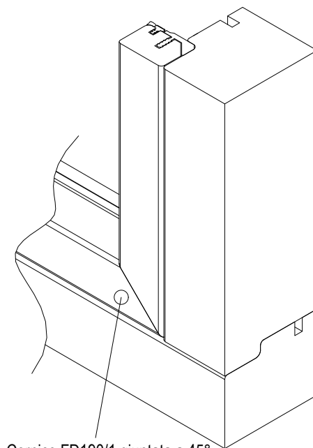
Cornice FD190/1 giuntata a 45°
