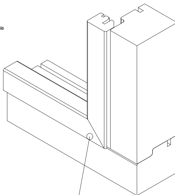
Cornice FD190/1 giuntata a 45°
