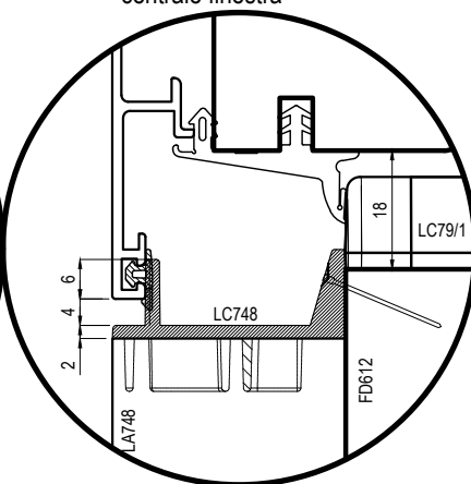
Sezione chiusura centrale finestra
